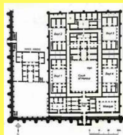
Ukhaidir - Palácio-fortaleza – 77 d.C.
